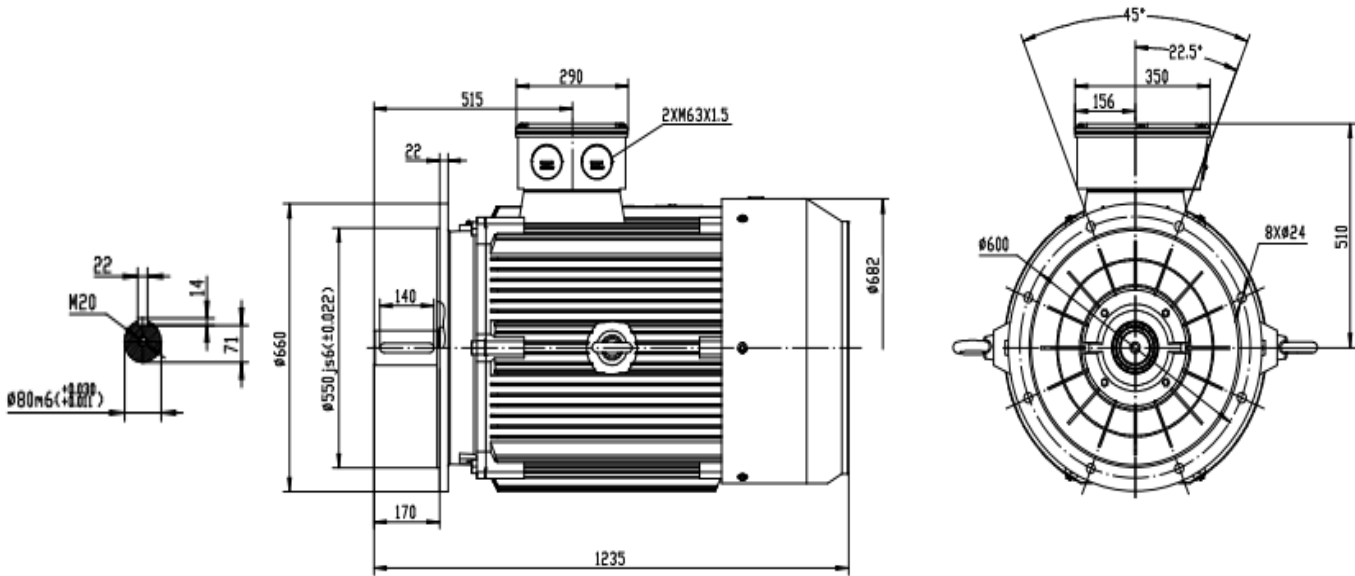
Typ / type IE3 SEV- 315S-8
