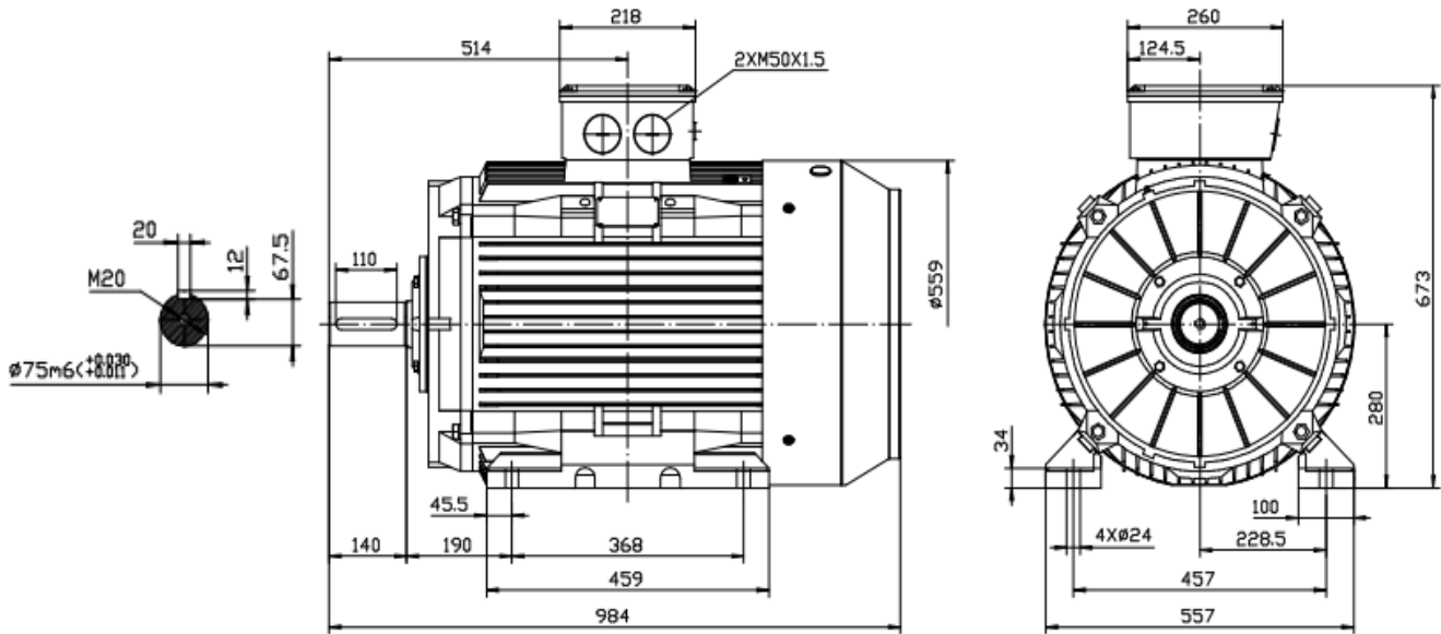
Typ / type IE3 SEV- 280S-6
