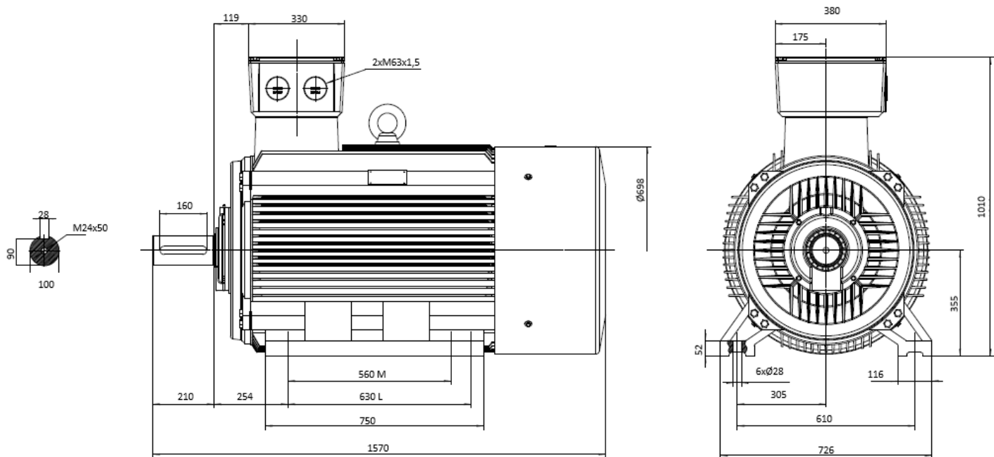
Typ / type IE4 SEV- 355M1-6
